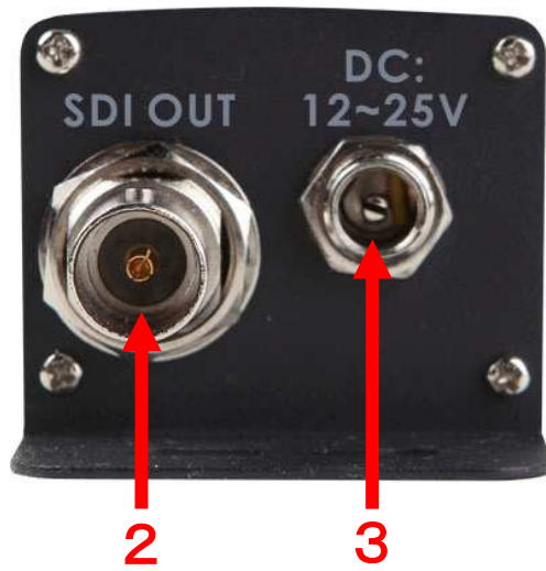
《後面パネル》
